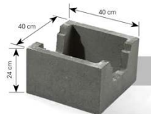
Pustak fundamentowy (z wpustem) symbol: D2 waga: ok. 30 kg
