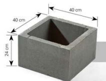
Pustak fundamentowy (pełny) symbol: D1 waga: ok. 33 kg
